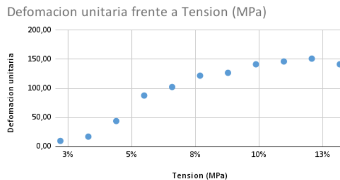
(a) Gráfica del ensayo de tracción de la barilla del aluminio ER4043 ensayo 1.
