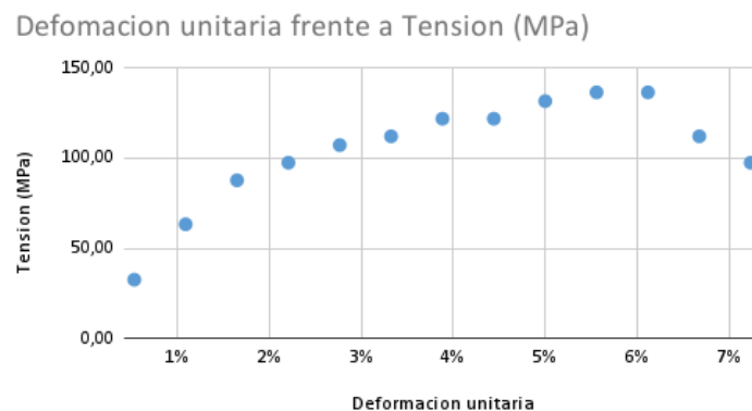
(b) Gráfica del ensayo de tracción de la barilla del aluminio ER4043 ensayo 2.
